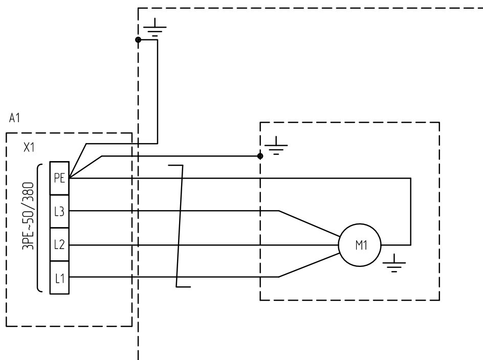
Рисунок 4. Электрическая схема завесы КЭВ-П9011А
