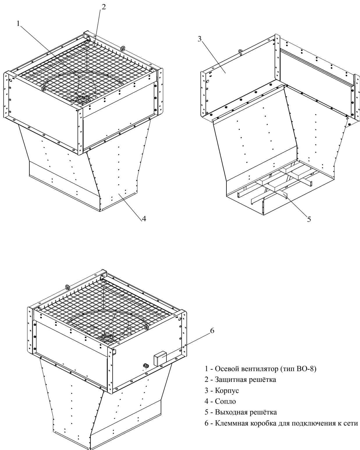
Рисунок 1. Основные узлы и детали завесы КЭВ-П9010А
