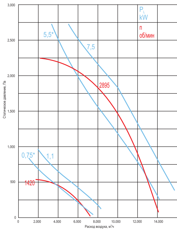
ВКР-4,5-ДУ-С-...
