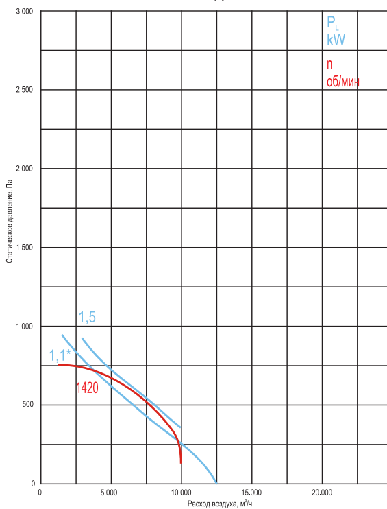
ВКР-5-ДУ-С-...
