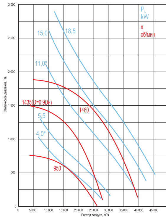
ВКР-8-ДУ-С-...
