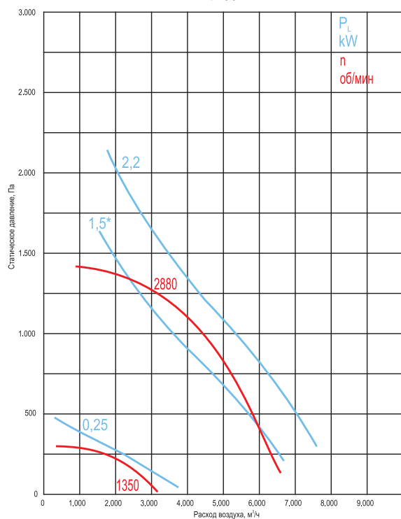
ВКР-3,5-ДУ-С-...
